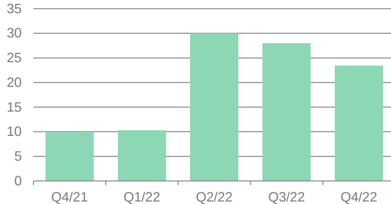
Kokonaisjalostusmarginaali, USD/barreli
